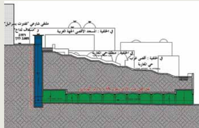
رسم بياني لنفقين مع مصعدين في حارة الشرف يوصلان الى ساحة البراق ٢٠٠٩/٣/٣
